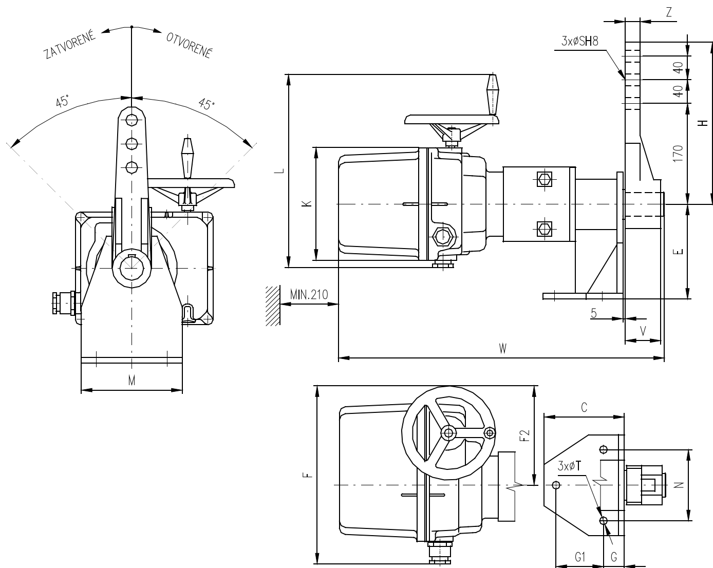
Hlavné rozmery
