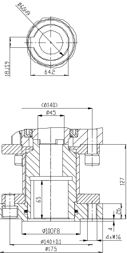
Kształt B1 \Shape B1\
