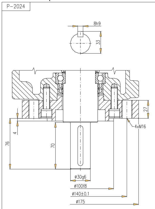
Kształt D \ Shape D
