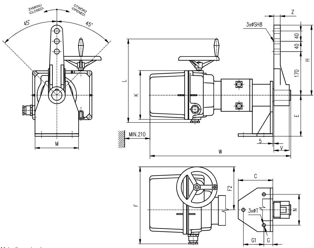
Główne wymiary \Main dimensions\
