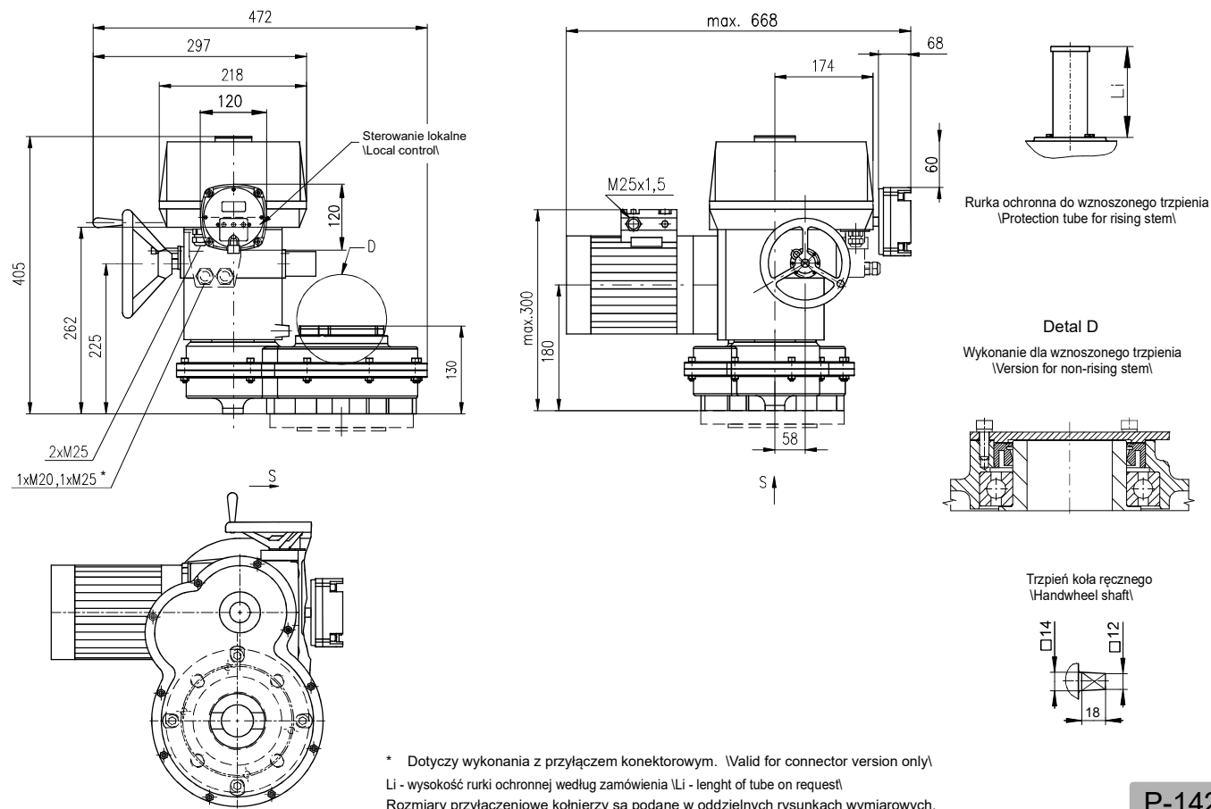
Rysunek wymiarowy MOR 3.5PA - w wersji z PROFIBUS/MODBUS \Dimensional drawings MOR 3.5PA - PROFIBUS and MODBUS versions\
