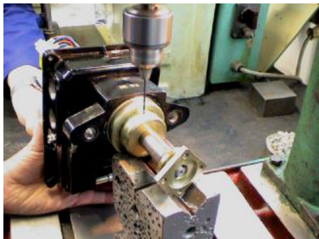
Montáž dorazovej trúbky do priamočiareho adaptéru, SN 5.3.2.2
